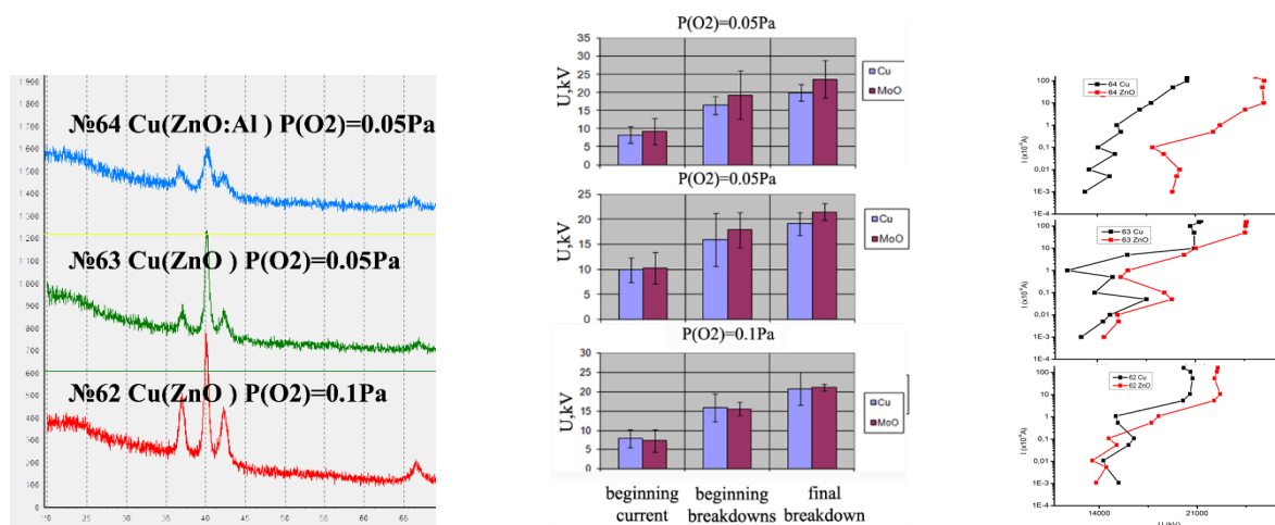
Рис3. Дифракційні спектри плівок \text{ZnO} та їх стійкість до пробоев
