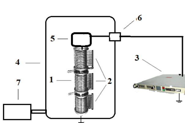
Рис. 1. Схема високовольтної структури. 1 – ПТ, 2 – резисторний дільник напруги (резистори SGT26), 3 – джерело високої напруги SL130P10 на 130 кВ [5], 4 – бак, 5 – кондуктор (високовольтний електрод), 6 – високовольтний ввід, 7 – система очищення повітря у баку.
