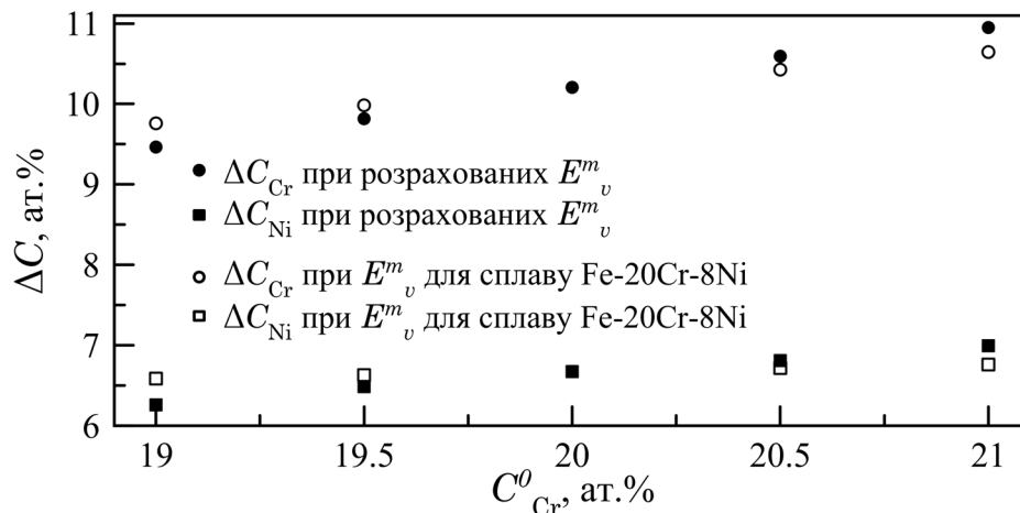
Рис. 1. Значення збіднення Cr та збагачення Ni для сплавів Fe-xCr-8Ni при енергіях міграції вакансій для сплаву Fe-20Cr-8Ni та розрахованих для кожного сплаву при x = 19; 19,5; 20,5; 21 .
