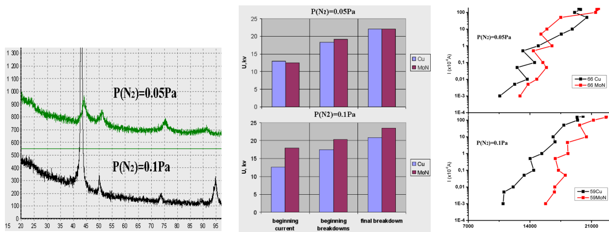
Рис. 2. Дифракційні спектри \text{Mo}_2\text{N} плівок, які відповідають зразкам з різною стійкістю до пробоев та результати вимірювань мідних зразків з плівками \text{Mo}_2\text{N} на стійкість до пробоев
