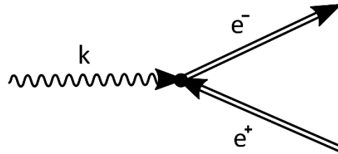
Рис. 1. Діаграма Фейнмана фотонародження e^- e^+ пари.
