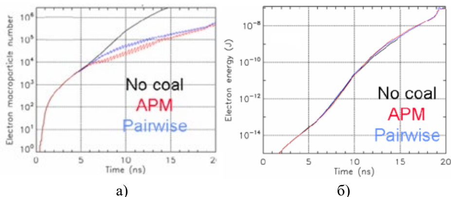
Рис.1. Результати моделювання 2D плазми методами: чорний – прямий метод, червоний – адаптивний алгоритм, синій – алгоритм попарного злиття [2]
