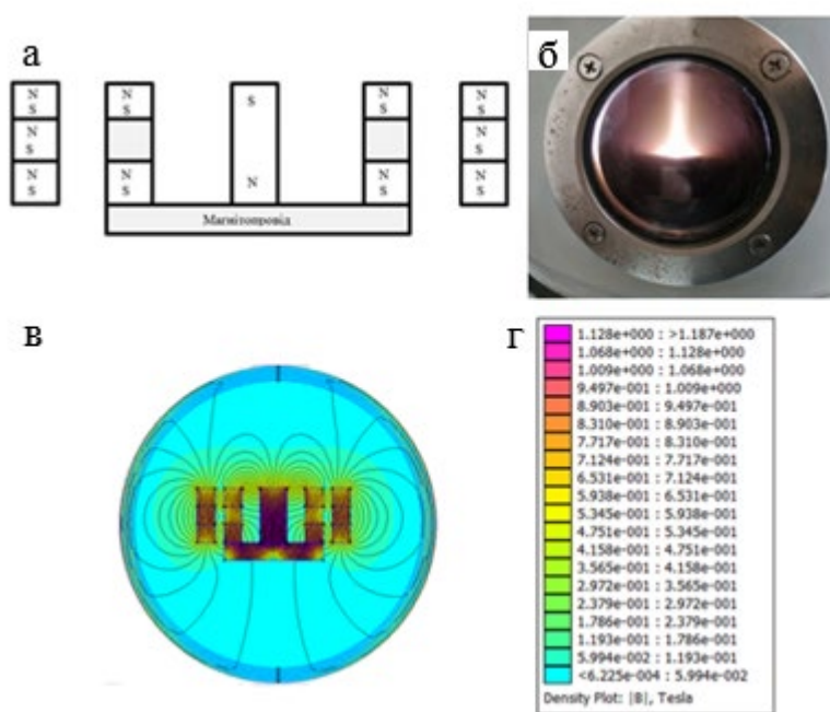
Рис. 1. Незбалансована МРС: а – схема магнітної системи; б – фото плазми магнетронного розряду; в – розподіл ліній індукції магнітного поля; г – шкала величини індукції магнітного поля
