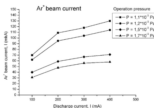
Рис. 3. – Залежність струму іонів Ar + від розрядного струму при різних значеннях тиску
